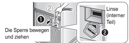
Luftansaugung für Staub/PM2,5-Sensor
